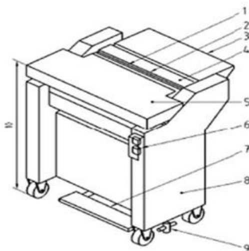
Figura 6 - Máquina aberta de descourear e de retirar a pele e a membrana
