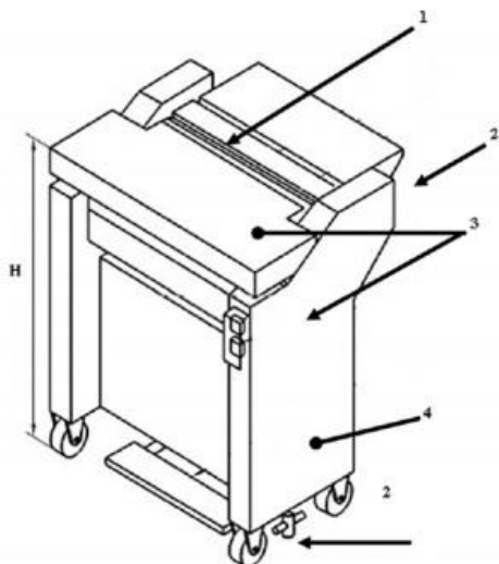
Figura 8 - Zonas de perigo da máquina aberta de descourear e retirar a pele e a membrana
