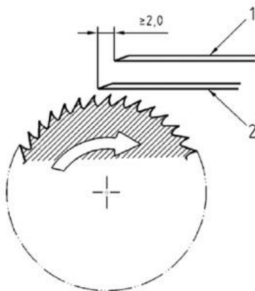
Figura 11 - Detalhe do dispositivo de lâmina dupla
