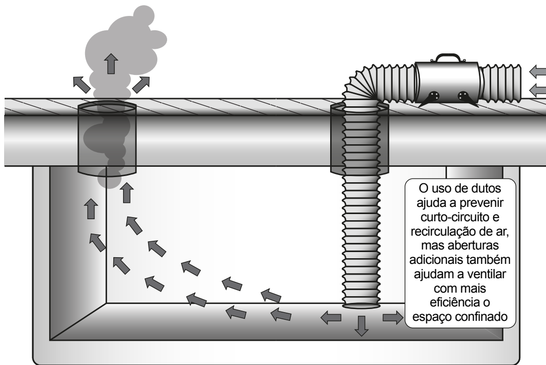
Figura B.8 – Sistema de ventilação por exaustão – Correção de curto-circuito de ar em espaços confinados
