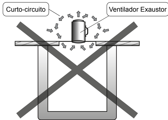
Figura B.4 – Sistema de ventilação por exaustão – Curto-circuito de ar em espaços confinados
