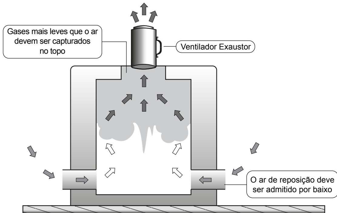
Figura B.2 – Sistema de ventilação de gases mais leves que o ar por exaustão
