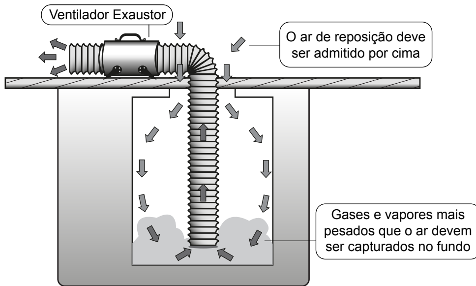
Figura B.1 – Sistema de ventilação de gases mais pesados que o ar por exaustão
