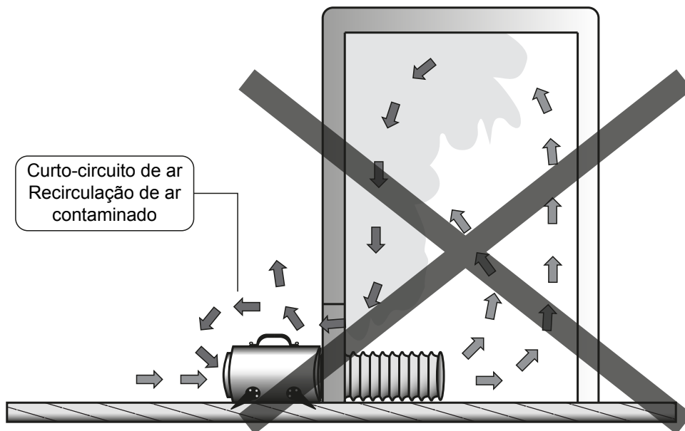
Figura B.7 – Sistema de ventilador por insuflação – Curto-circuito de ar – Recirculação de ar
