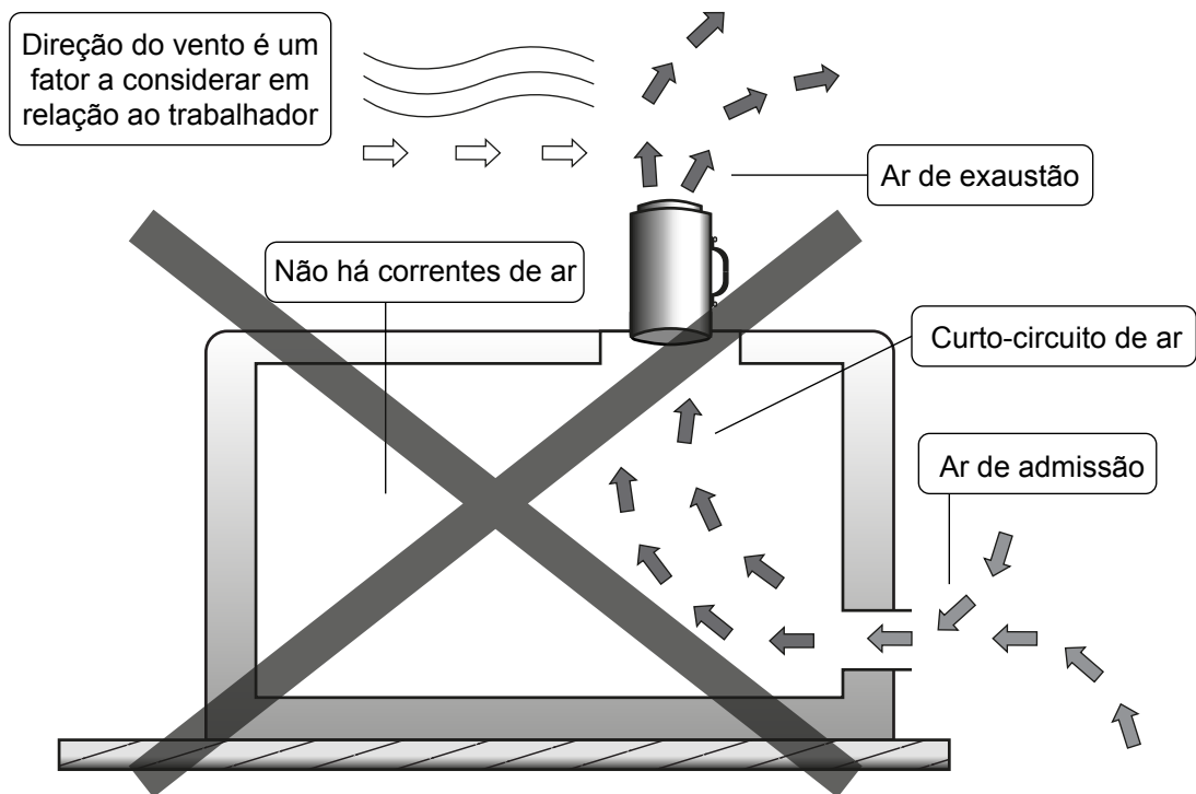
Figura B.6 – Sistema de ventilação por exaustão – Curto-circuito de ar em espaços confinados
