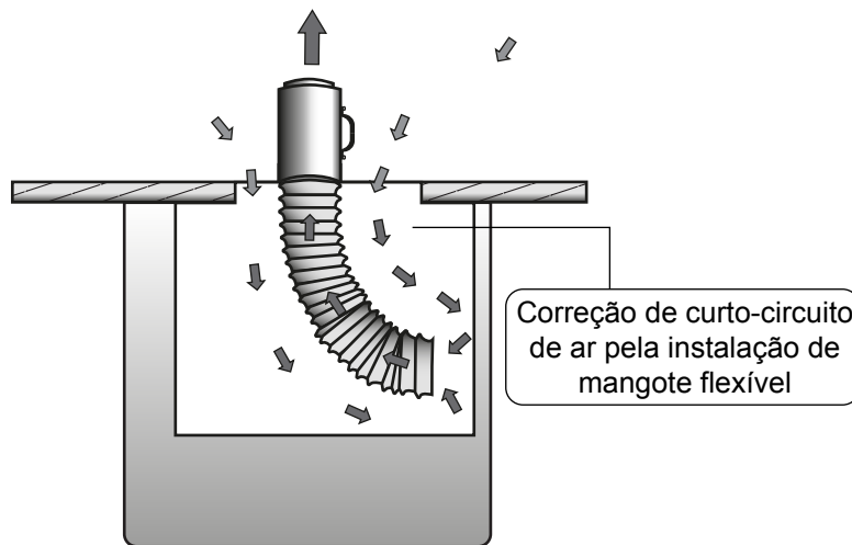
Figura B.5 – Sistema de ventilação por exaustão – Correção de curto-circuito de ar em espaços confinados
