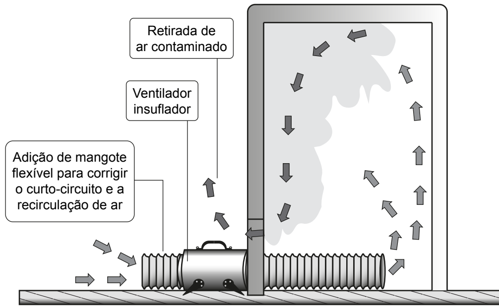
Figura B.10 – Sistema de ventilação por insuflação – Correção de curto-circuito de ar pela instalação de mangotes flexíveis
