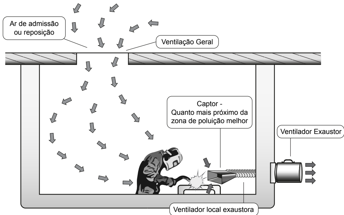
Figura B.3 – Ventilação local exaustora em espaços confinados – Controle dos fumos de solda na fonte contaminante
